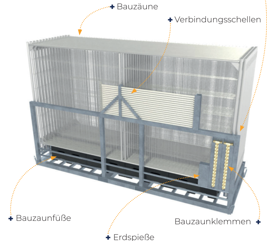
Transportgestell für Absperrgitter
