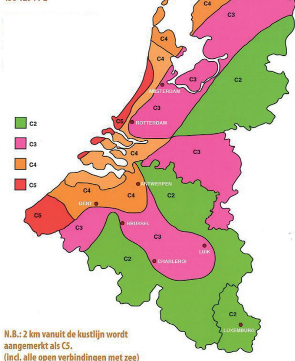
Invloed van klimaat en luchtgesteldheid volgens NEN-EN-ISO 12944-2
